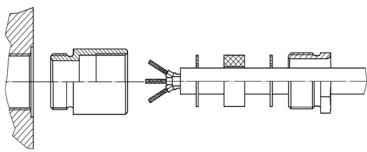
Montage Verschraubung SMR:
