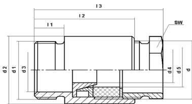
Montage Verschraubung SMR-EMV:
