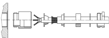
Montage Verschraubung SMR-EMV:
